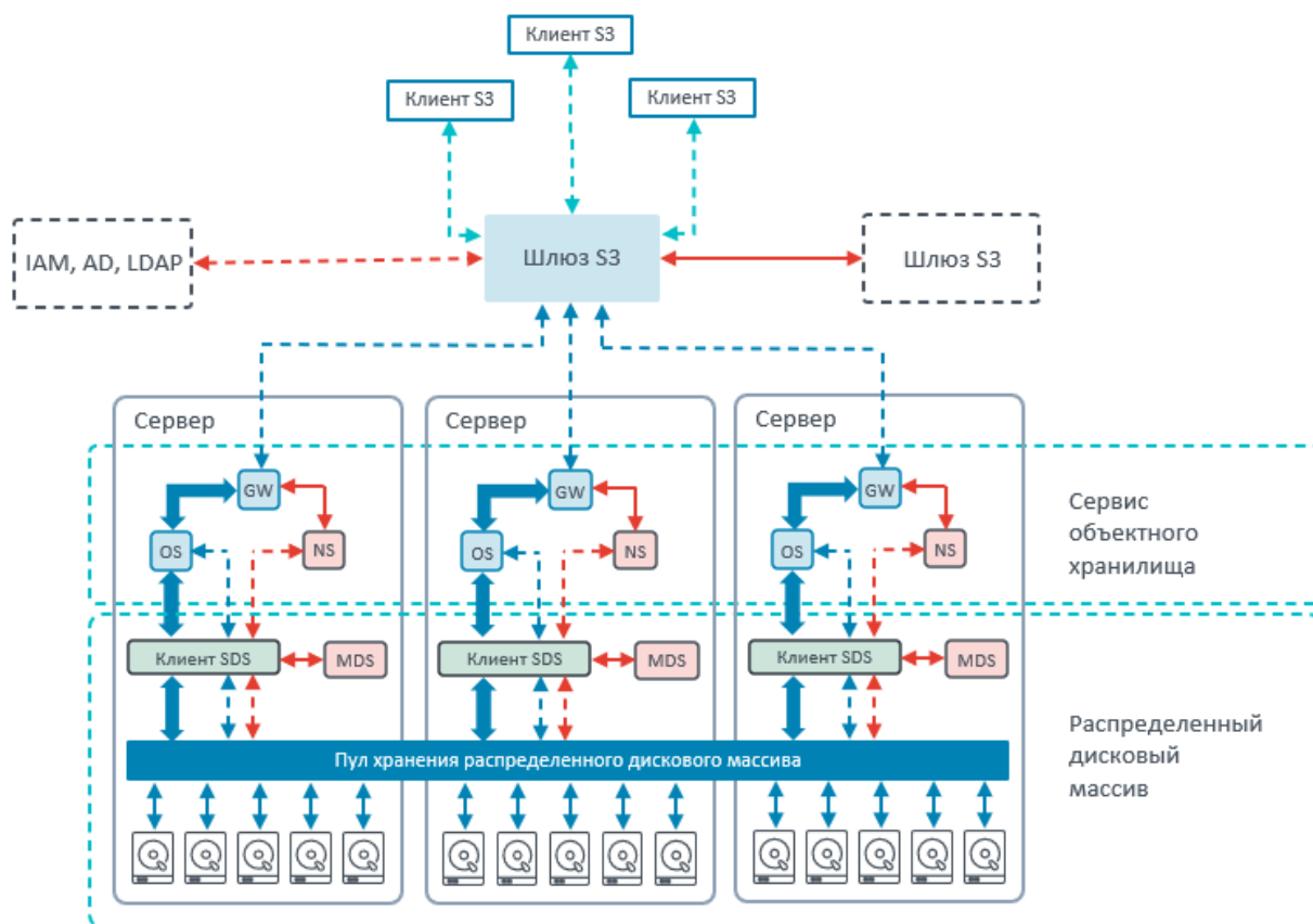
Рисунок 2. Архитектура Машины хранения данных (Схема внутренней коммутации)
