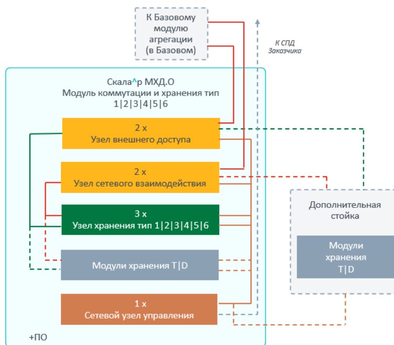
Рисунок 7. Схема модуля коммутации и хранения
