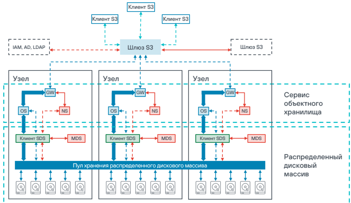
Рисунок 2. Архитектура Машины хранения данных (Схема внутренней коммутации)
