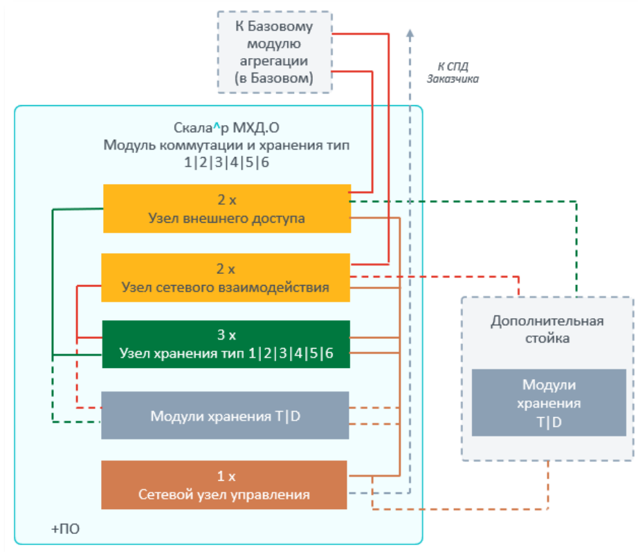
Рисунок 7. Схема Модуля коммутации и хранения
