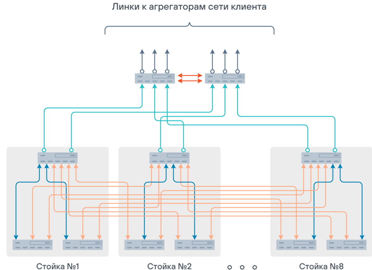
Схема внутренних соединений Leaf-Spine с увеличением скорости при горизонтальном масштабировании
